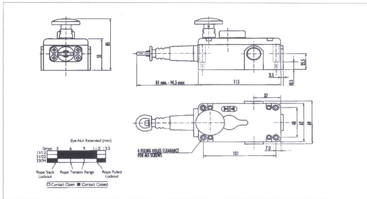
Fig. 2 Dimensions
