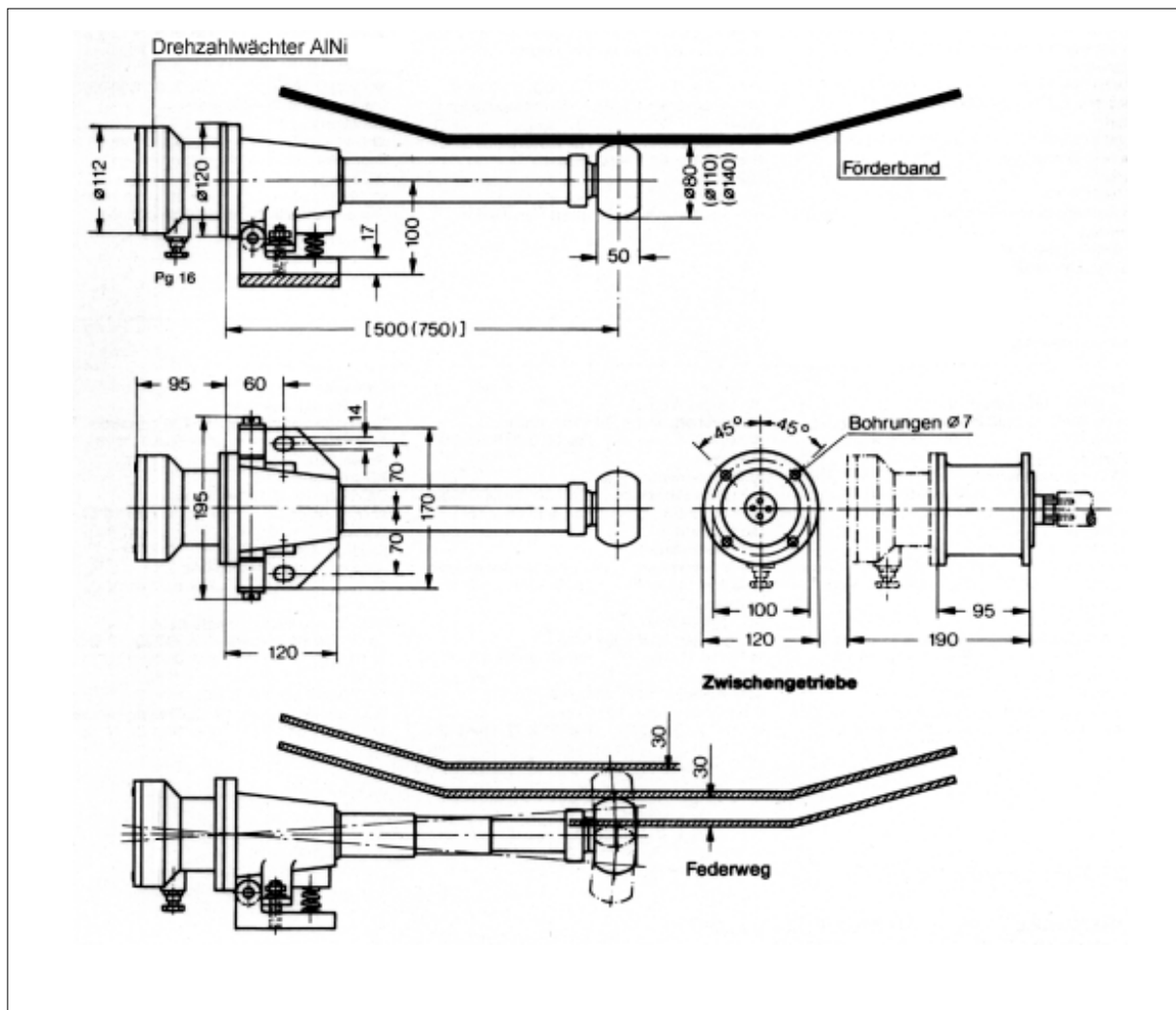
Maßbilder
