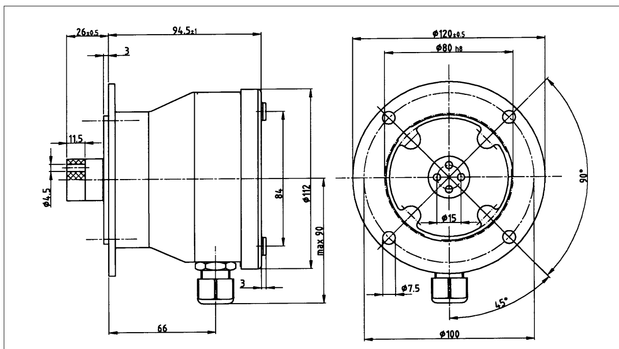
Maßzeichnung des Drehzahlwächters Al-Ni 6
